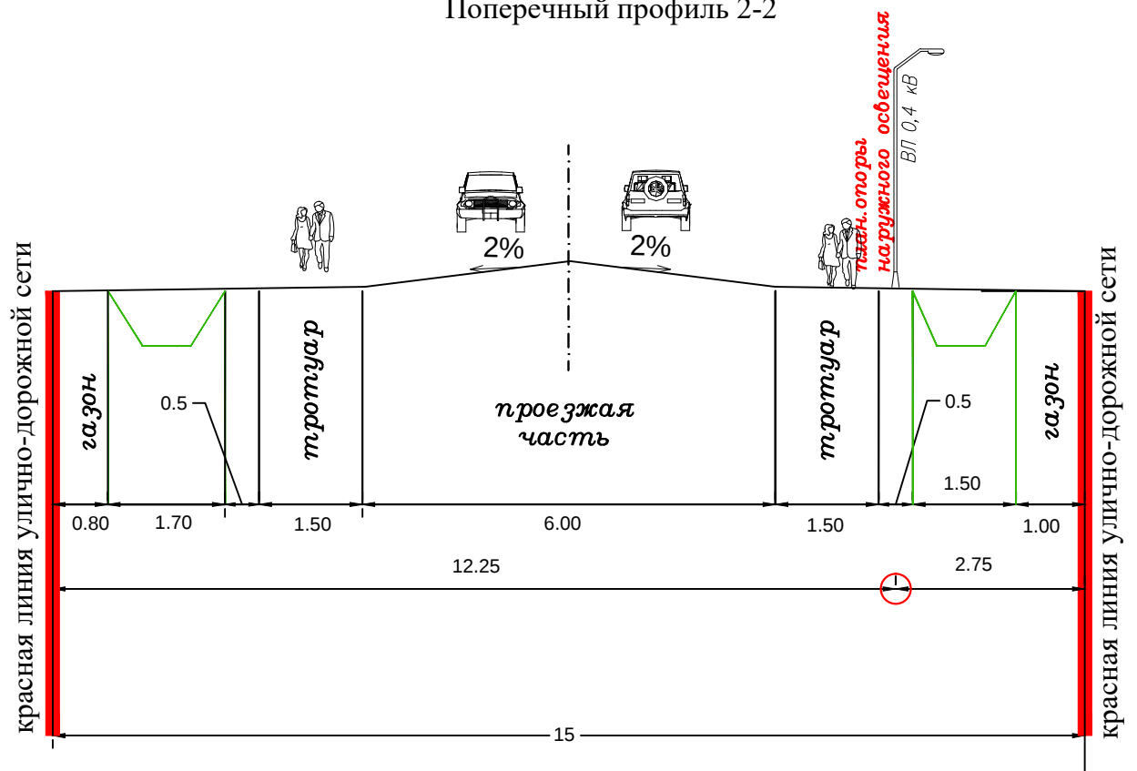
Поперечный профиль 2-2
